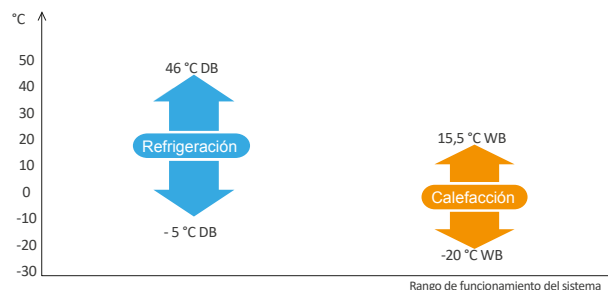
Rango de funcionamiento del sistema
