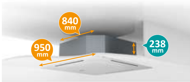
Cassette de 4 vías
